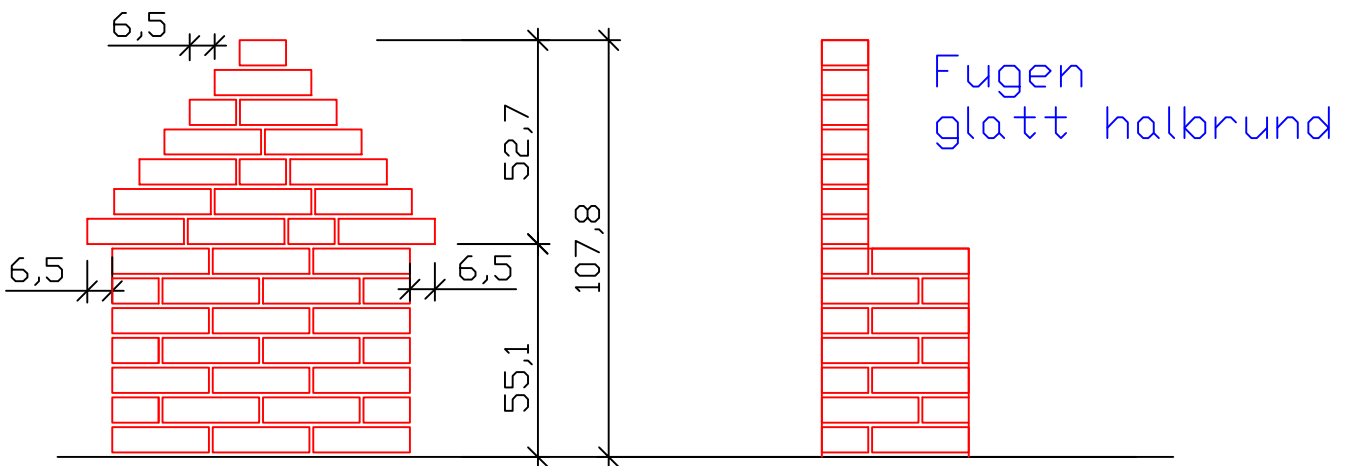
Vorderansicht
