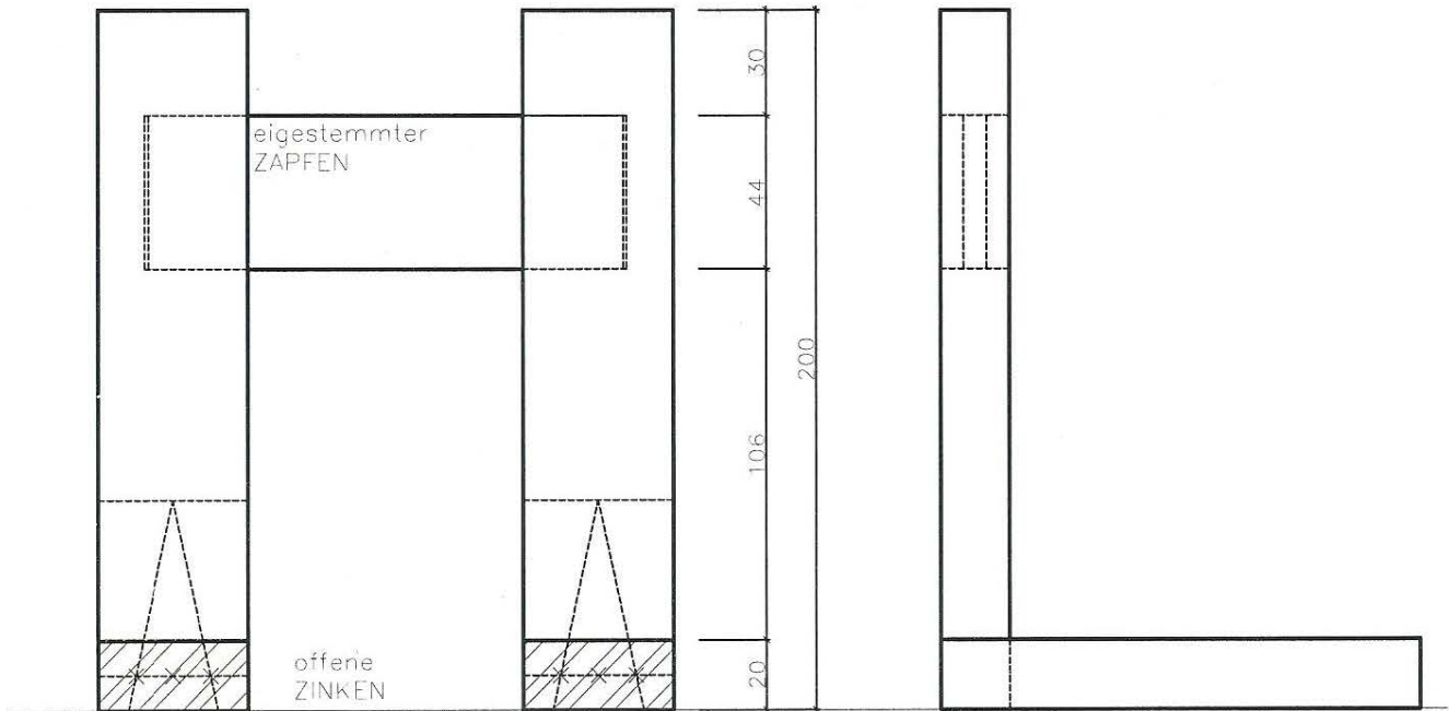
KREUZRISS
