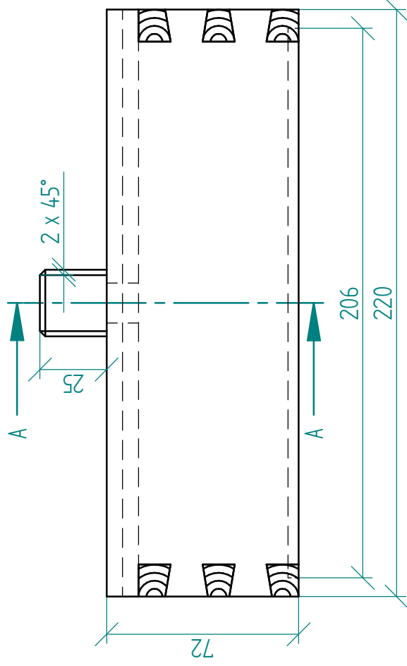
Aufriss
