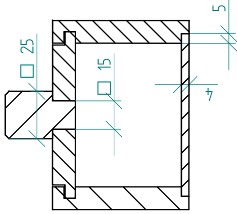
Schnitt A-A
