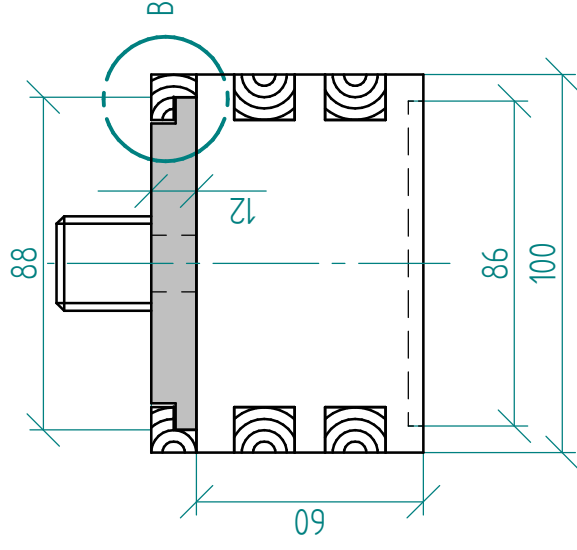
Kreuzriss
