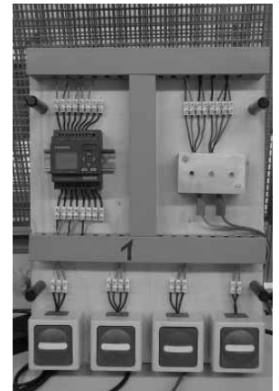
Grundplatte
